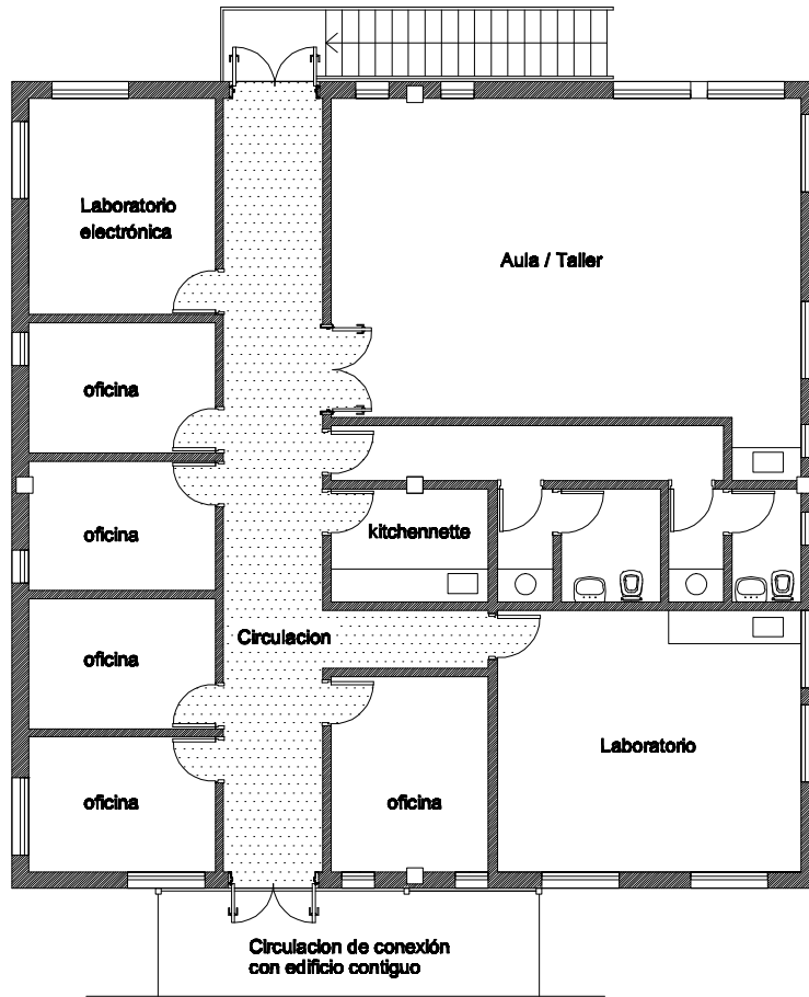
PLANTA ALTA
